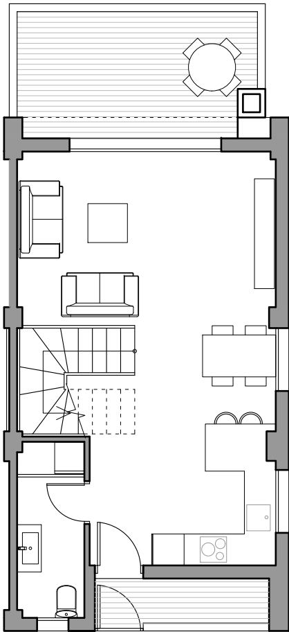
PLANTA BAJA
